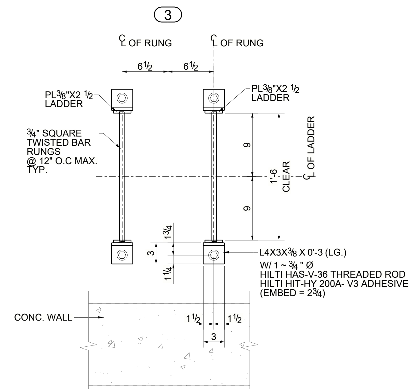
SECTION 1A - 1A
