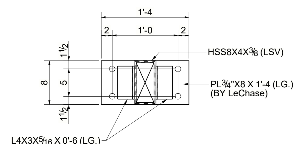
SECTION 1A - 1A
