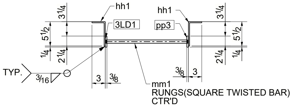
D - D
