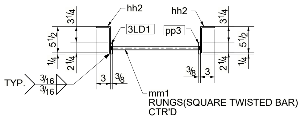
E - E
