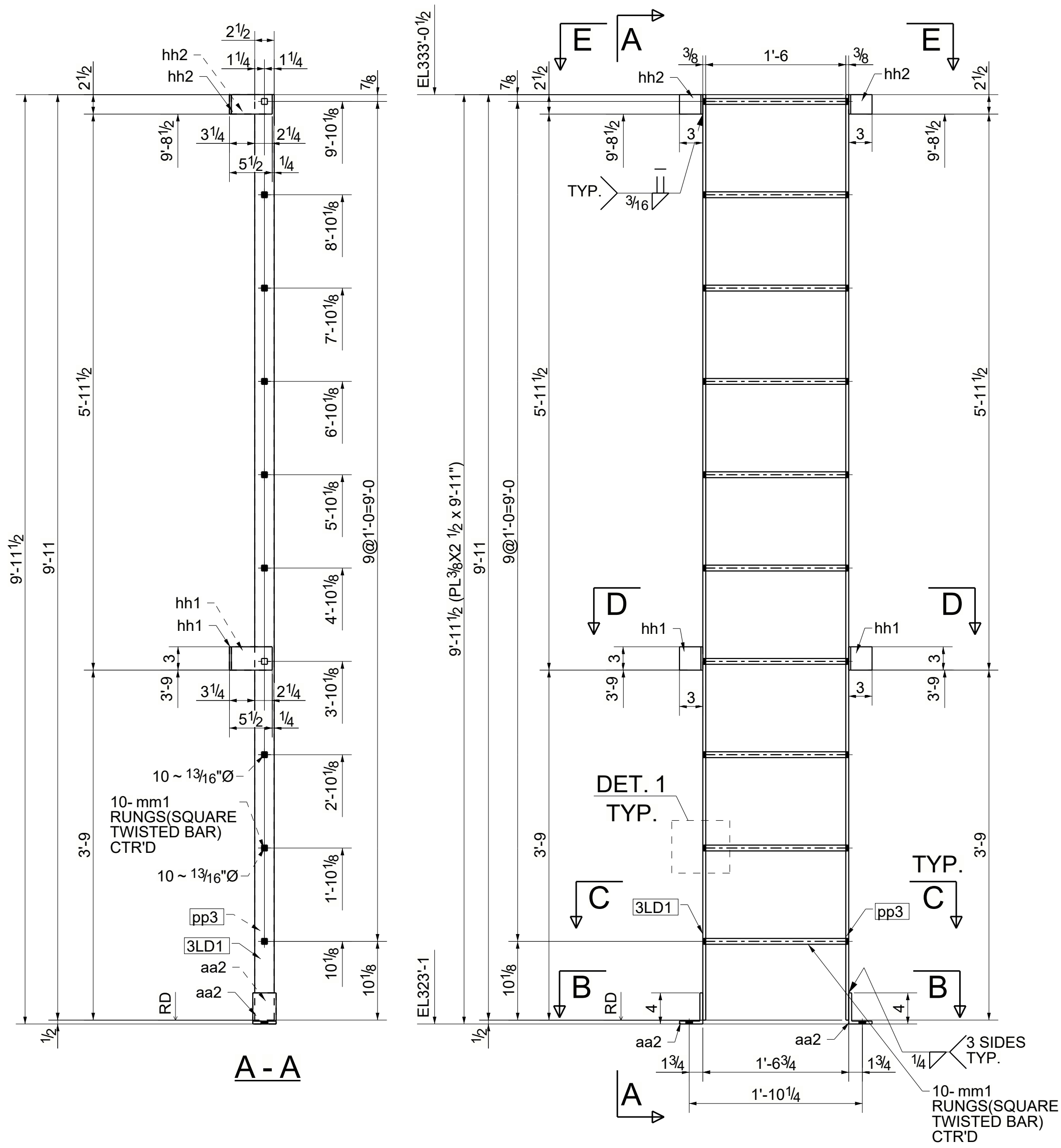
2 - LADDERS - 3LD1
